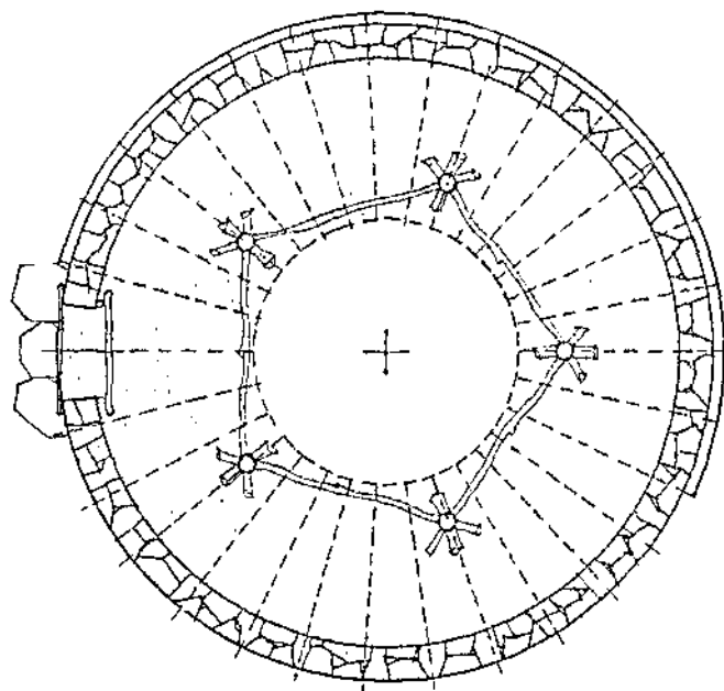
Tloris prve značilne oblike ovčnjakov.
