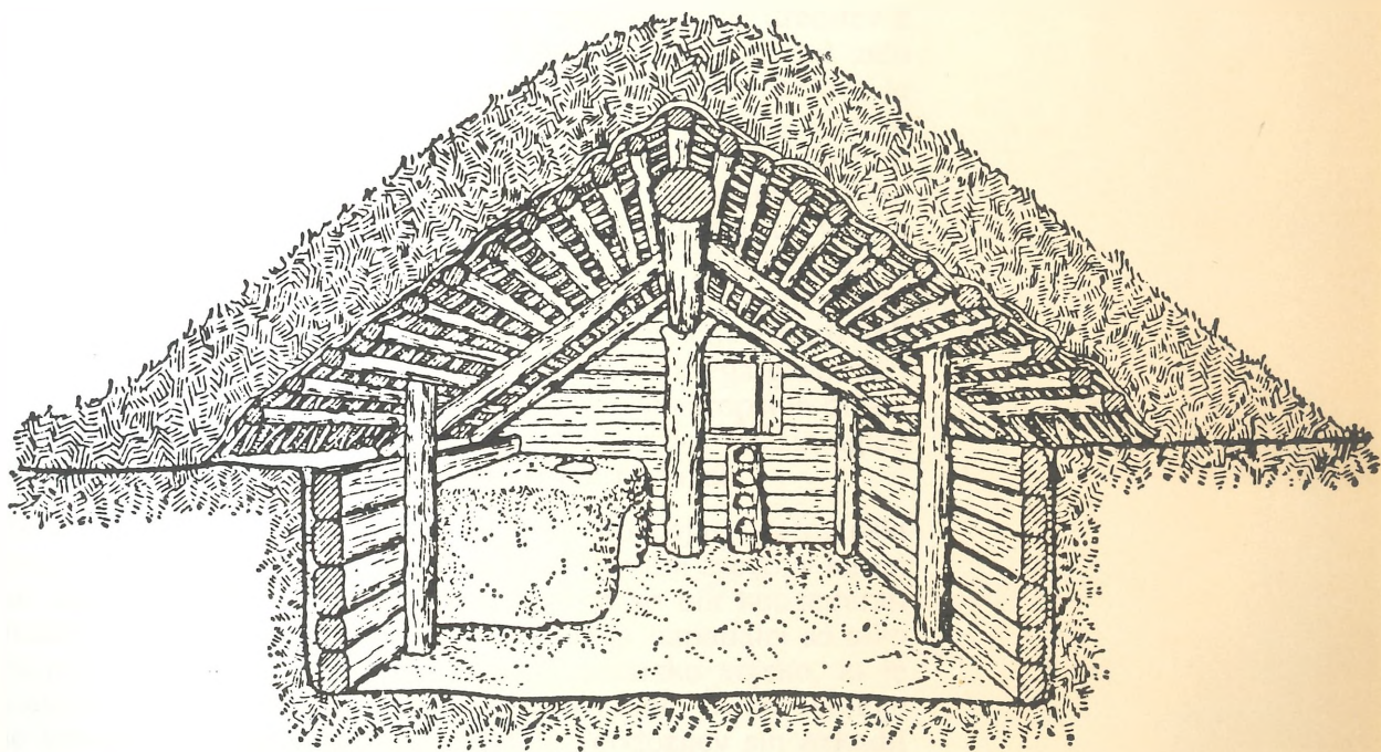
Rekonstrukcija slovanske kočē – polzemljanke (6., 7. stol.)
