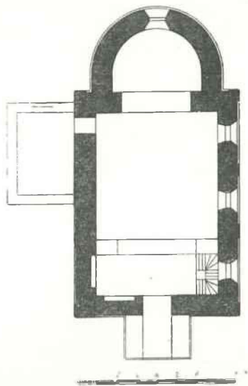
Sl. 2. Tloris cerkve v Domanjševcih
