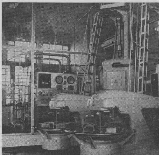
Polnilnica za polnjenje sterilnih mlečnih izdelkov
