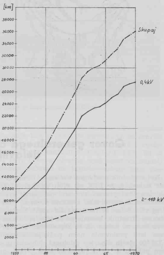
Dolžine distribucijskih omrežij v km
