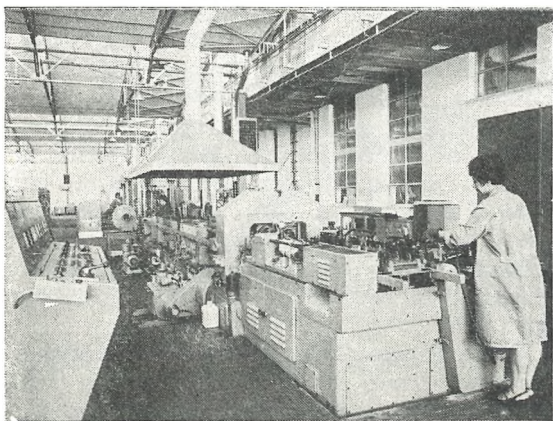
Nova linija za izdelovanje konservnih škatel z zmogljivostjo do 9000 kosov na uro, postavljena v obratu Zalog, specializiranem za proizvodnjo konzerv
