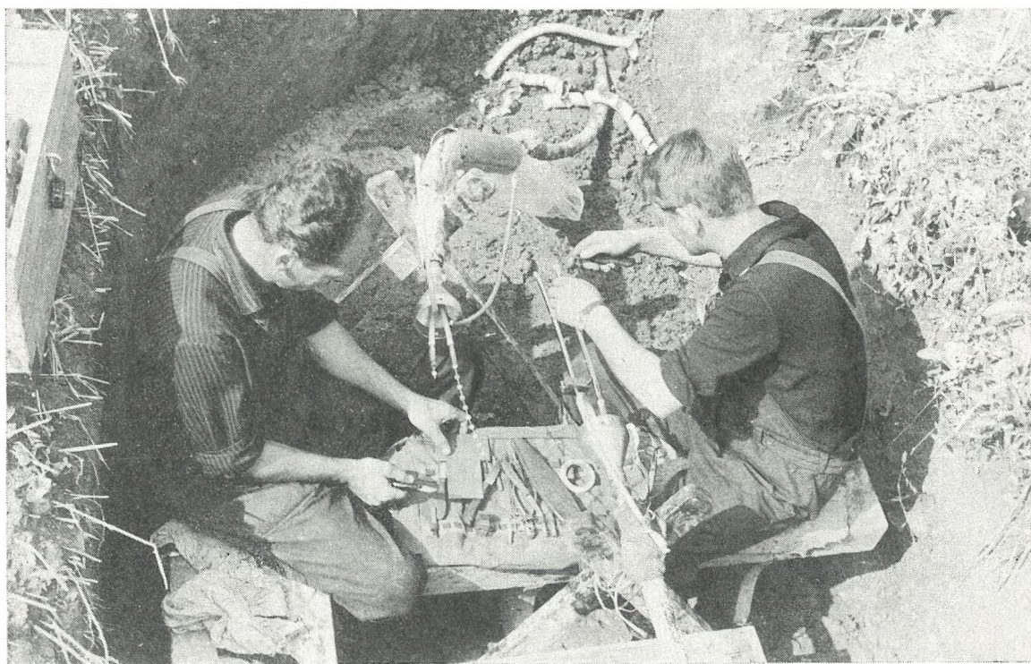
Montažna dela na medkrajevnem kablu.
