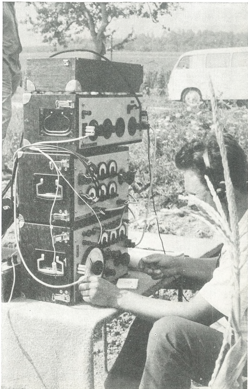
Kapacitivna izravnava medkrajevnega kabla.
