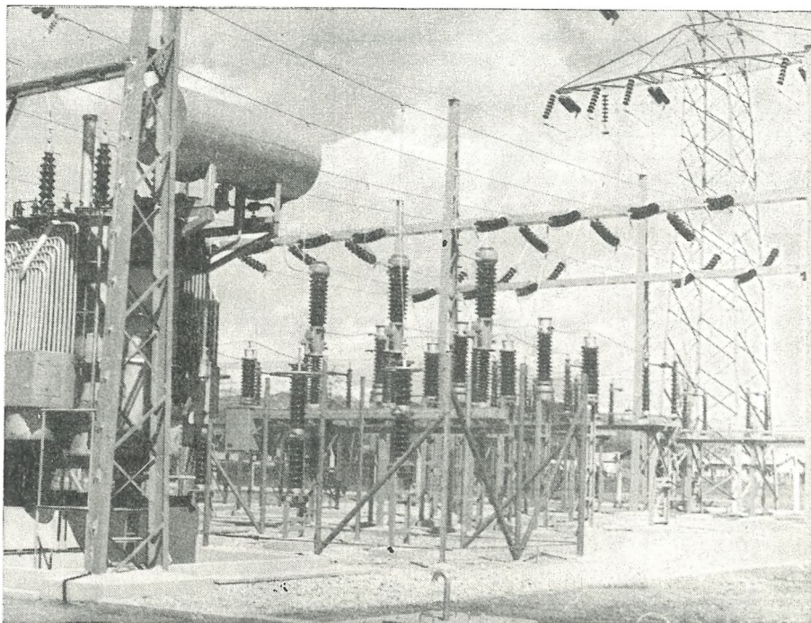
RTP Ljubljana-Siška 110 kV stikalo
