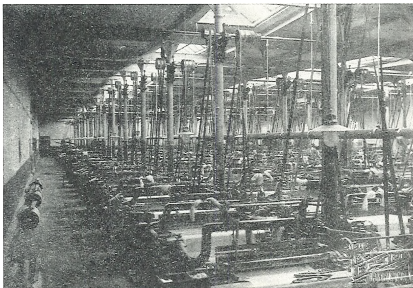
Dvorana tkalnice z 272 stavitvami v tekstilni tovarni v Trzinu leta 1922
