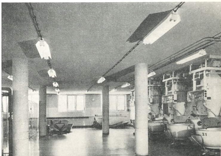
Moderna pekarska mešalnica testa
