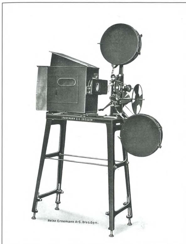
Filmski projektor Ernemann »REX« (vir: internet)
