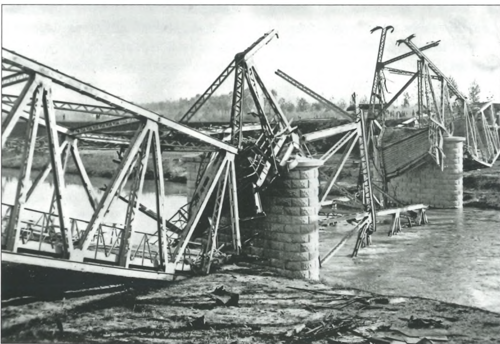
Most v Motti di Livenza, ki so ga ob umiku uničili Italijani. (fototeka Goriškega muzeja)
