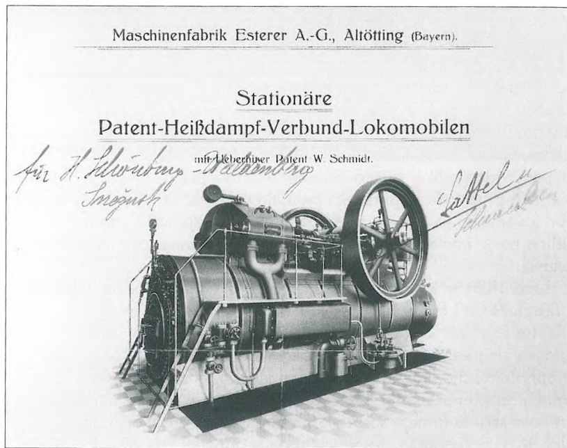
Slika lokomobile, ki so jo montirali na žagi Marof za žaganje lesa, kot spremni dokument ob dostavi stroja na Snežnik. (Kopijo originala hranita Majda Obreza Špeh in Janez Špeh.)
