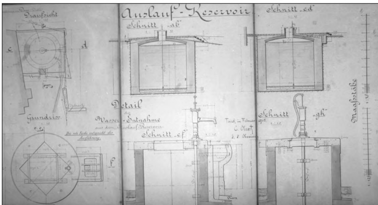
»Predelan načrt« za vodnjak v vasi. Z rdečo so označene spremembe, ki jih je bilo potrebno izvesti ob napeljavi vodovoda. Z rdečo je zarisan tudi predviden betonski obok cisterne, ki pa ni bil izveden (SI PAK, KP 633, š. 472).
