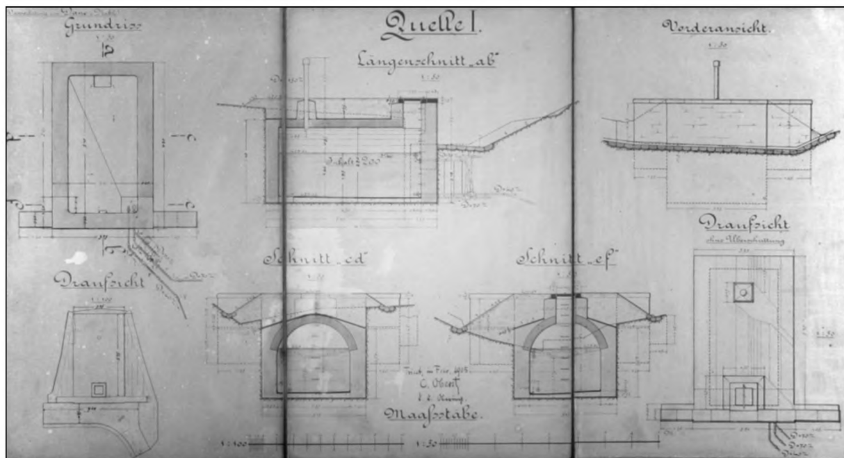
Načrt za izvedbo zbiralnika I, Ta guranjem študencu (SI PAK, KP 633, š. 472).
