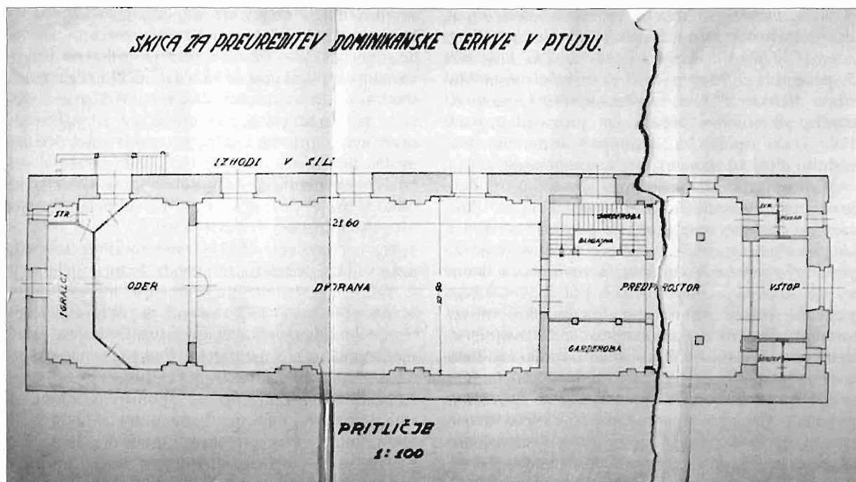
Načrt za gledališko dvorano v nekdanji cerkveni ladji dominikanskega samostana (ZAP, MOP, šk. 266, ovoj 273/26)
