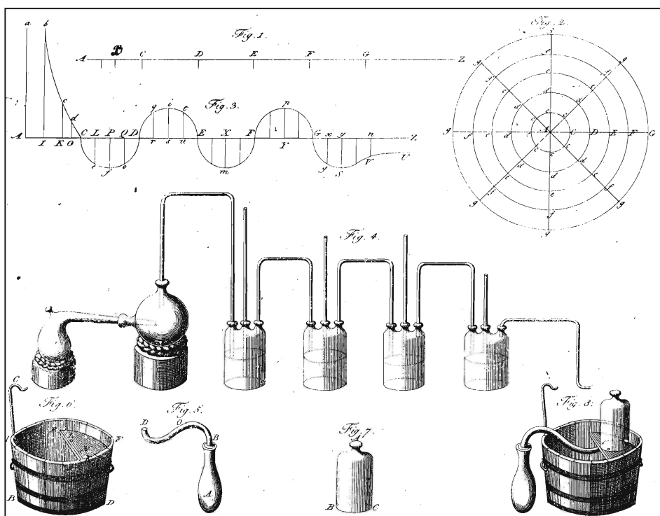
Slike iz Ambschellove mehanike, tiskane leta 1807. Fig. 1-3: Boškovičeva sila.
