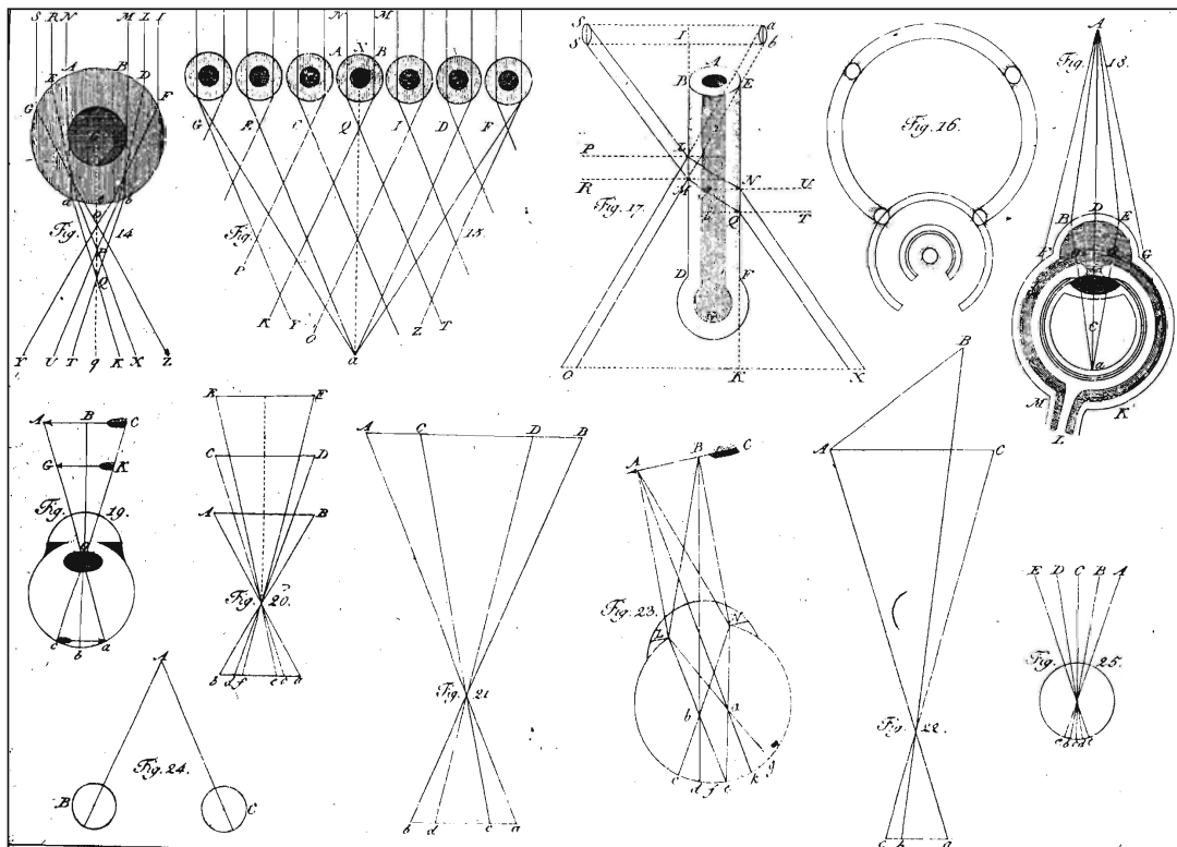
Slike iz Ambschlllove II knjige o optiki iz leta 1807. Tab. II: delovanje očesa, last avtorja.
