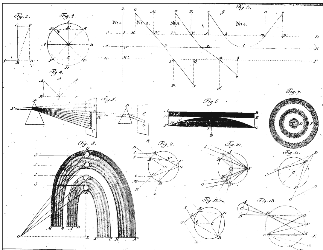
Slike iz Ambschlllove II knjige o svetlobi iz leta 1807: Tab. I: odboj in lom svetlobe z mavrico na Fig. 8.
