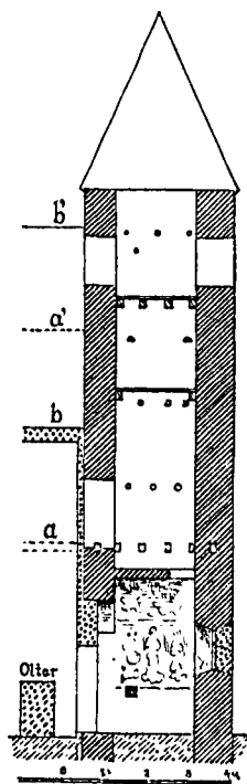
Sl. 3. Presek stolpa od zapada proti vzhodu.
