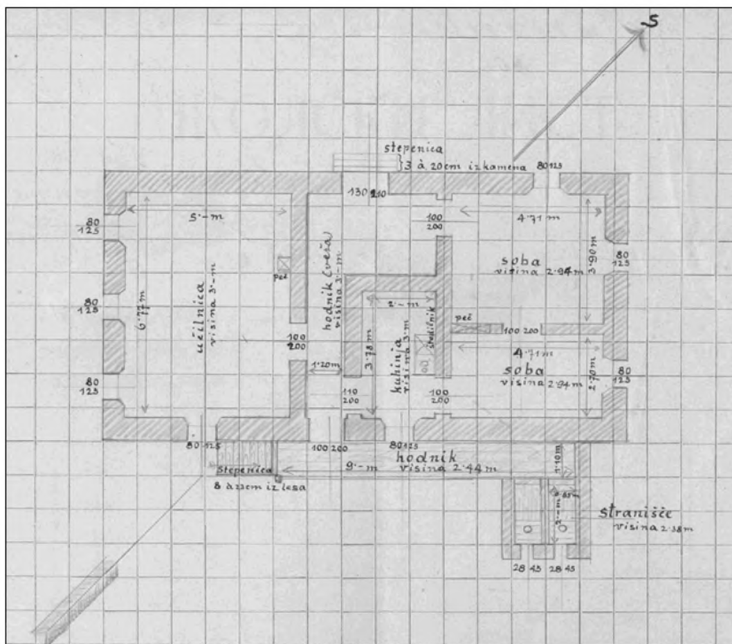
Tloris šolskega poslopja na Smuki z učilnico in učiteljskim stanovanjem, kakršno je bilo že za časa prvega učitelja Franza Kuglerja (SŠM, arhivska zbirka, šolski list OŠ Smuka, okraj Kočevje, 1929).
